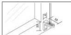
Spannwinkel 15.0104 transparent
