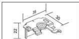
Wand- und Deckenträger 15.5372 silber
