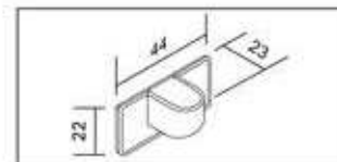
Magnethalter 15.1113 2 Stück weiß
